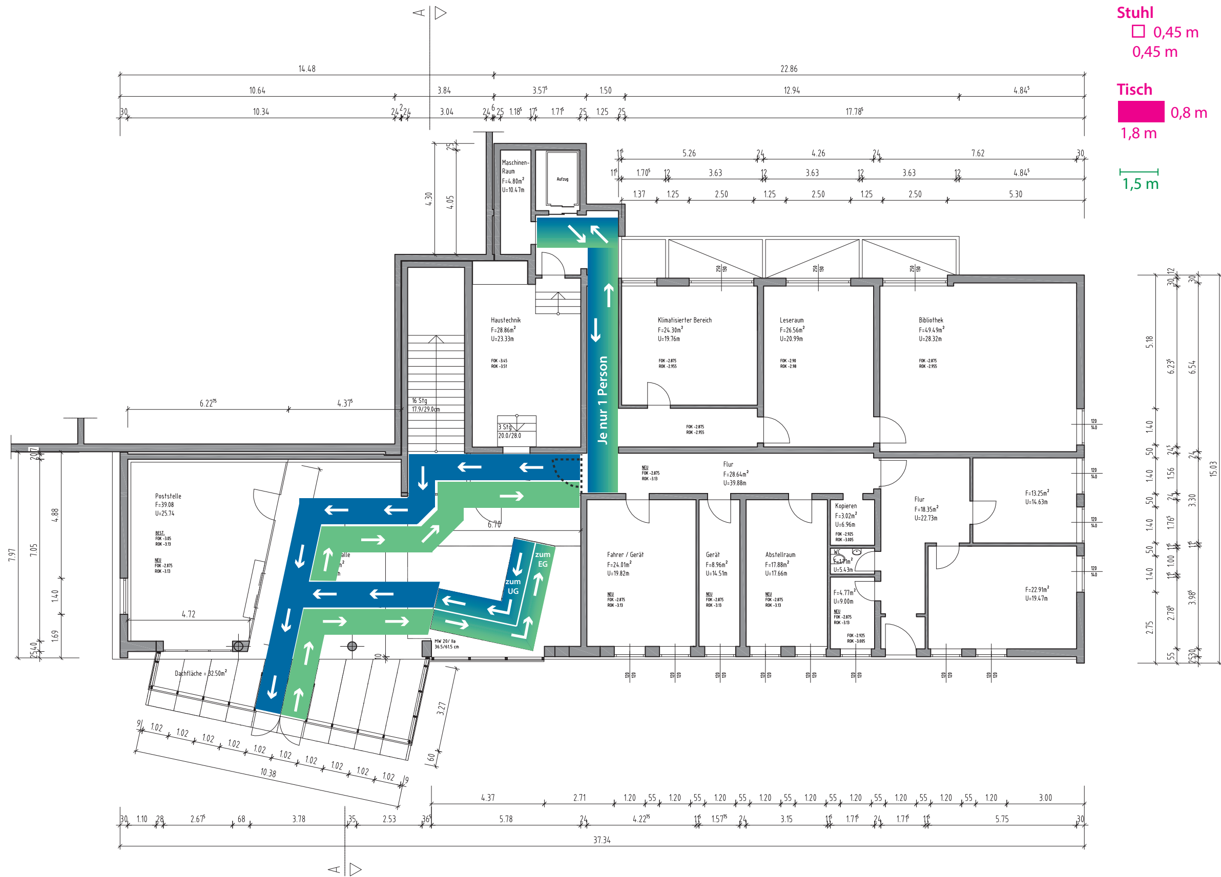
Untergeschoss
